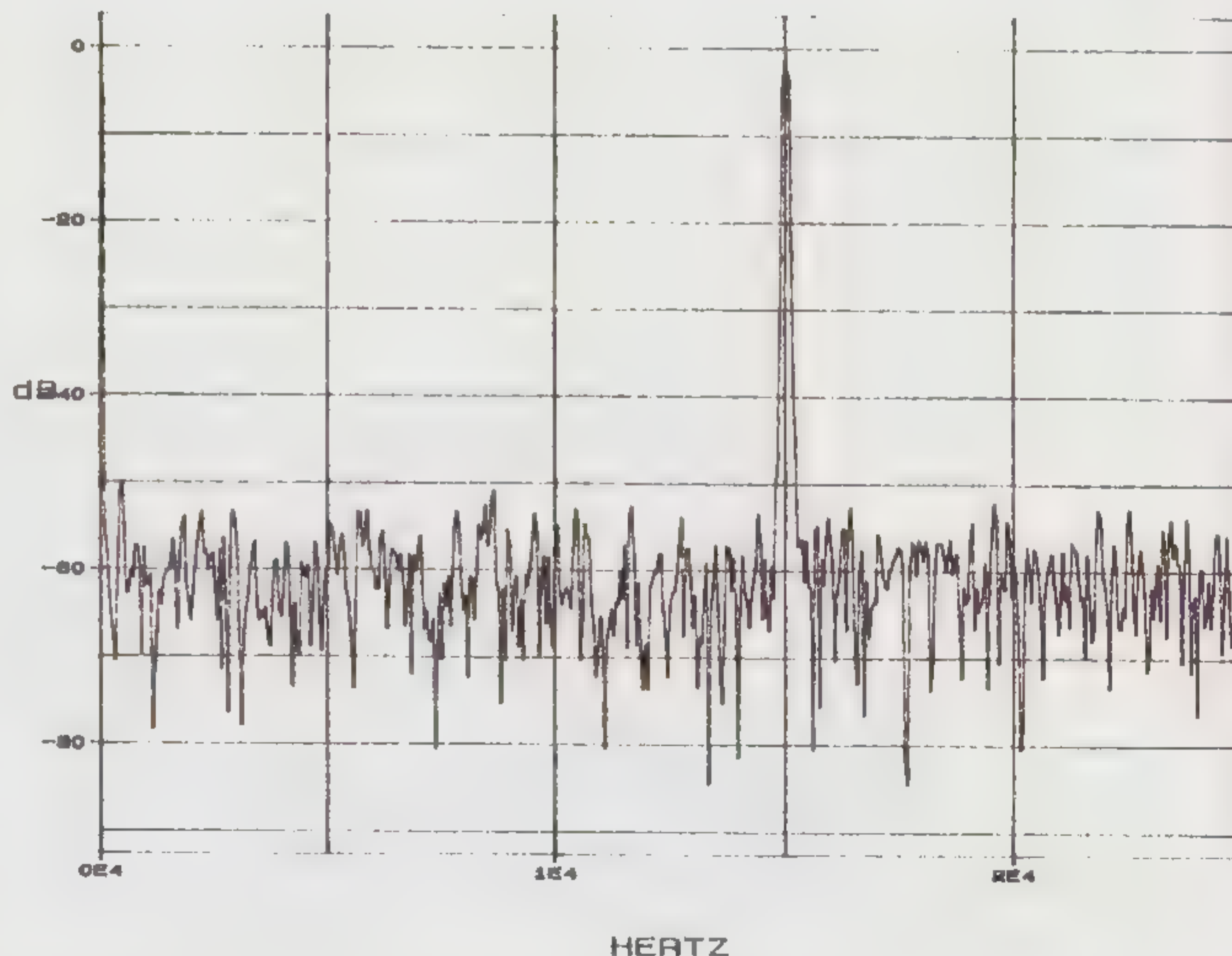
Figuur 8. De LF-Intermodulatie gemeten aan de versterkeruitgang
